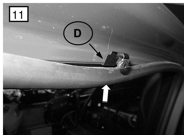
Der Halter wird unter dem Gummi auf das Blech gesteckt / The holder is under the rubber put on the sheet metal
